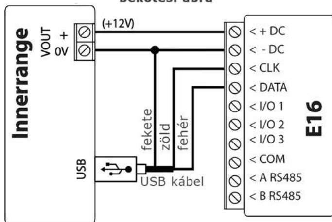
Innerrange Inception központ bekötési ábra
