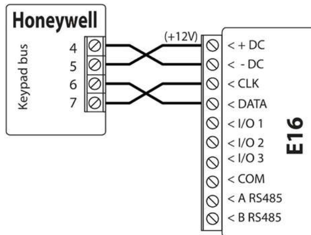
Honeywell Vista-20, Vista-48 központ bekötési ábra
